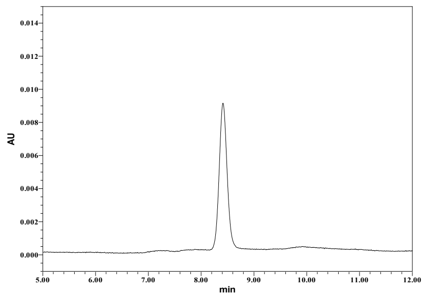
图A.1 1,1'-磺酰基二(4-氯苯)标准溶液的液相色谱图
